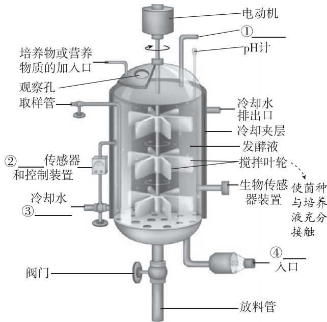
发酵罐示意图
